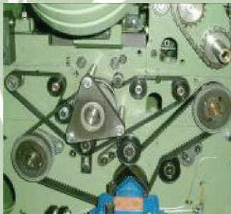
時規皮帶傳動系統
