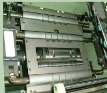
軟式刀模磁性滾輪
